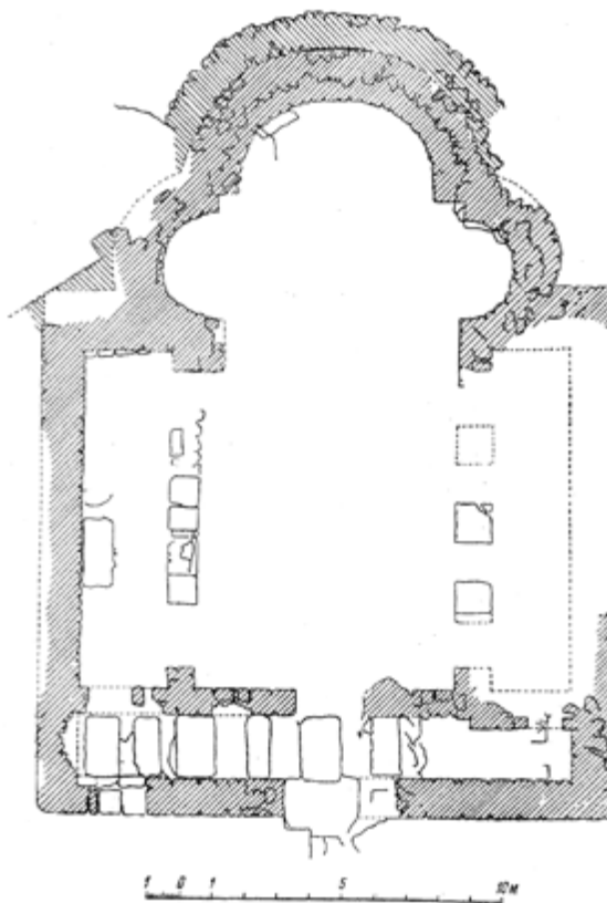
План Базилики Крузе (А.Л. Якобсон, 1959)
